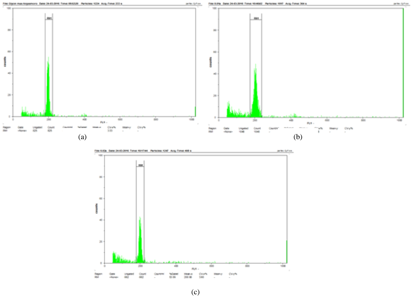
Gambar 1. Hasil analisis derajat ploidi dengan menggunakan flow cytometry pada daun muda tanaman (a) kedelai Anjasmoro kontrol, (b) kedelai Anjasmoro perlakuan kolkisin 0,01%, dan (c) kedelai Anjasmoro perlakuan kolkisin 0,02%
